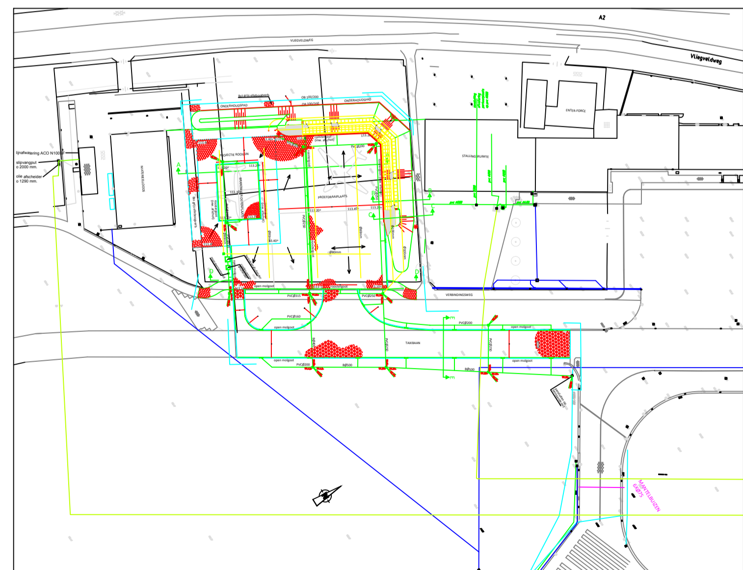
DETAIL 1 riolering afsputplaats
