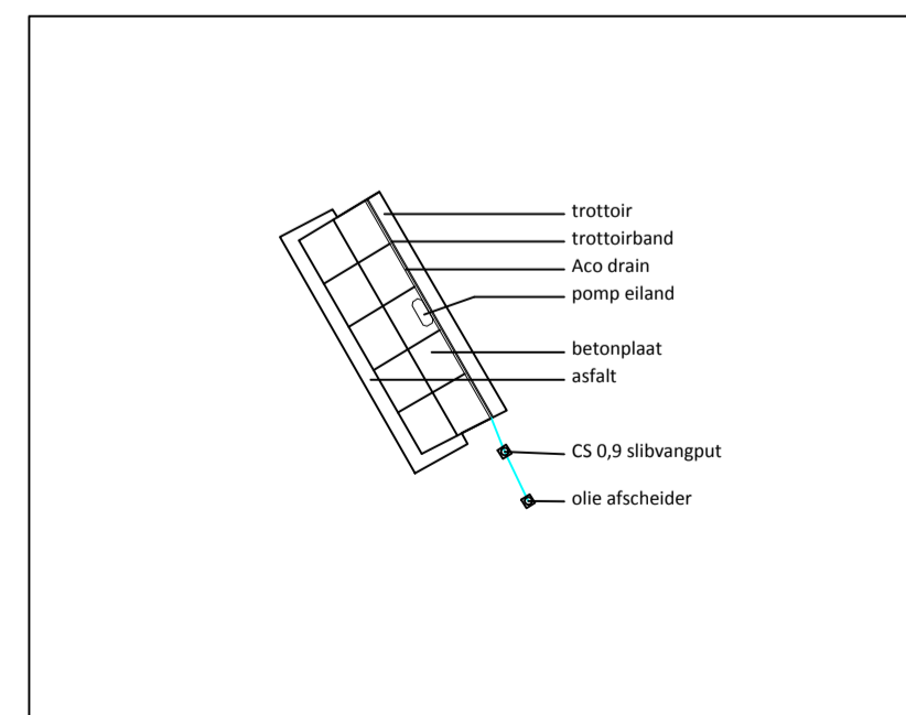
DETAIL 4 tankplaats Shell
