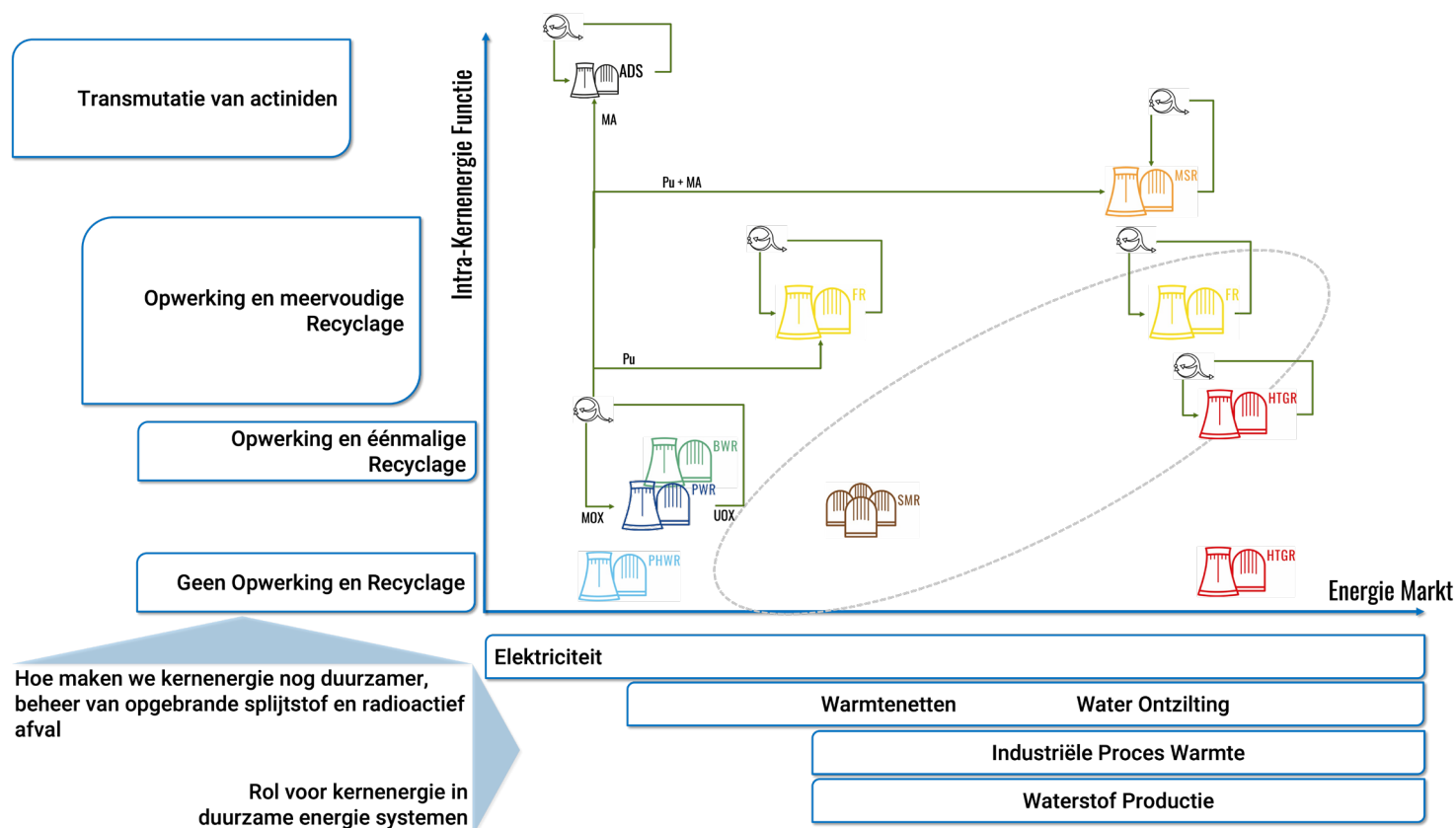
Figuur III.2 Overzicht van de kernenergie-opties in ontwikkeling
