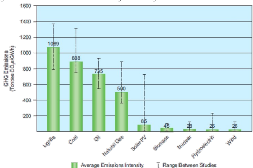
Figuur C.1 GHG-emissies voor energie-technologieën
