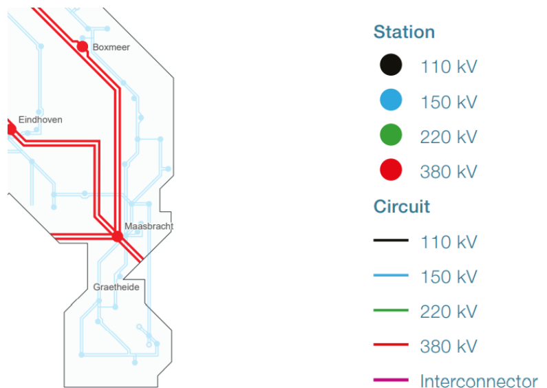
Figuur V.3 Netaansluitingen provincie Limburg
