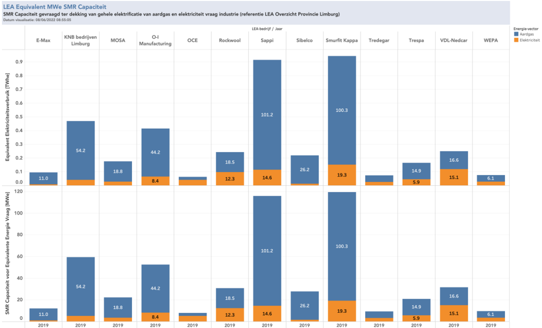
Figuur IV.5 LEA bedrijven equivalent elektriciteitsverbruik
