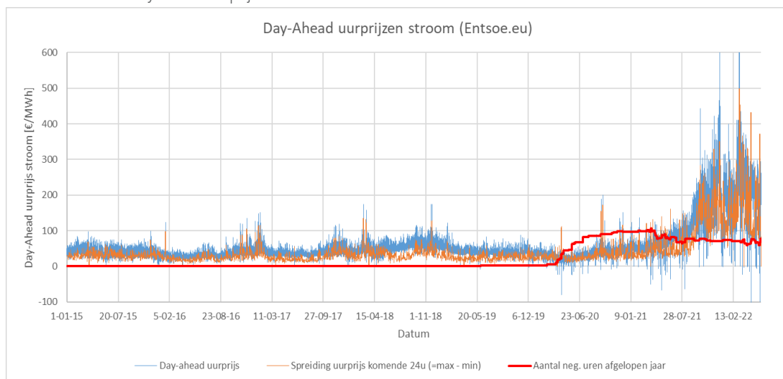
Figuur II.5 Evolutie van day-ahead elektriciteitsprijzen met duidelijk een toenemende spreading van de prijzen
