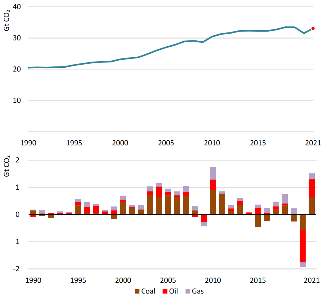
Figuur II.2 Globale energie-gerelateerde CO 2 emissies 1990-2021 en wijziging in CO 2 -emissies per type brandstof
