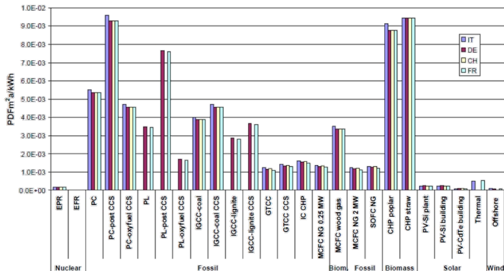
Figuur C.3 PDF criterium voor elektriciteitsproductie
