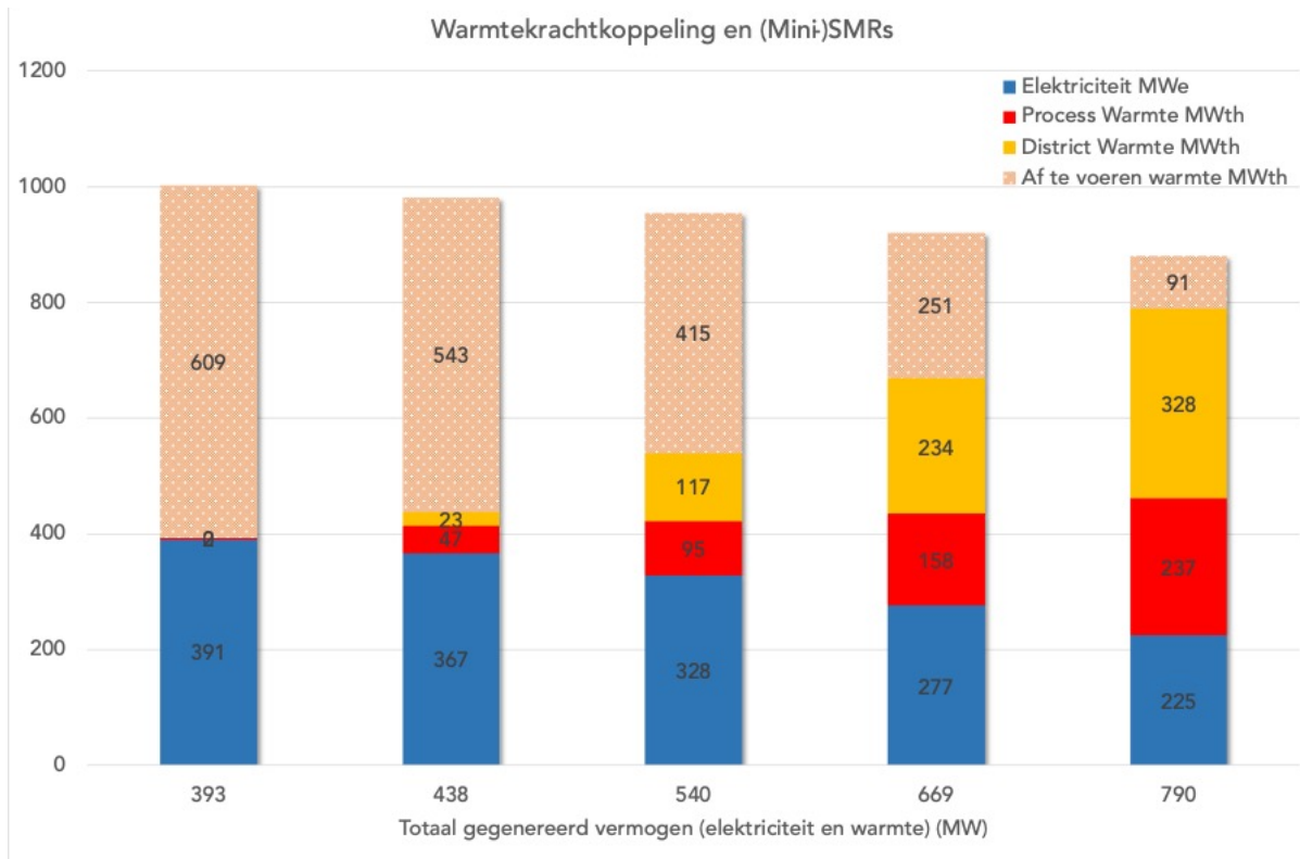
Figuur IV.7. SMRs en warmtekoppeling mogelijkheden naar maximaal gebruik van elektriciteit en warmte
