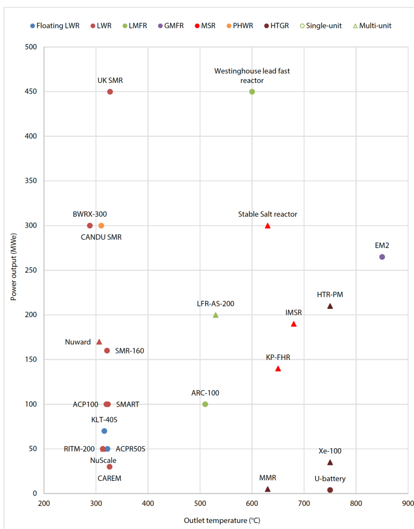
Figuur III.3 Eén van de mogelijke klassificaties van SMRs
