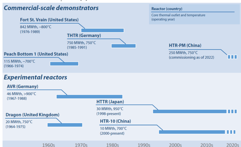
Figuur III.13 HTGR experimentele reactoren en demonstratie-plants [1].
