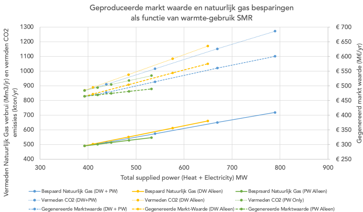
Figuur IV.8 Overzicht analyse van marktwaarde en bespaarde natuurlijk gas en CO2 emissies door warmtekrachtkoppeling van (Mini-)SMRs
