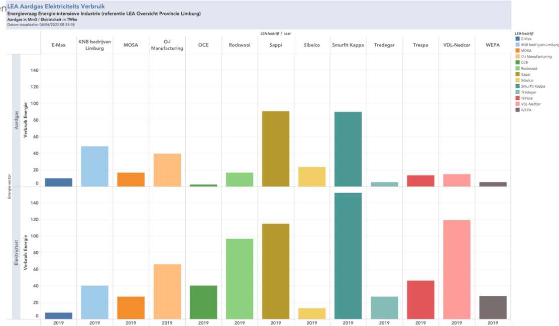
Figuur IV.4 LEA-bedrijven aardgas en elektriciteitsvraag in 2019
