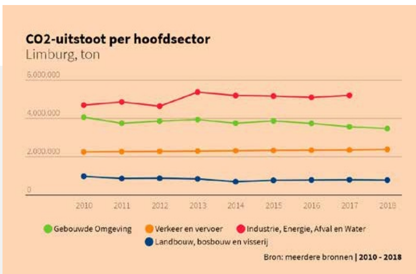
Figuur I.1 Jaarlijkse CO 2 -uitstoot in Provincie Limburg per hoofdsector gedurende de periode 2010-2018
