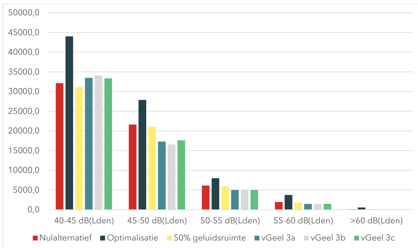
Figuur 6.1 Aantal woningen in Zuid-Limburg per geluidsbelastingscontour
