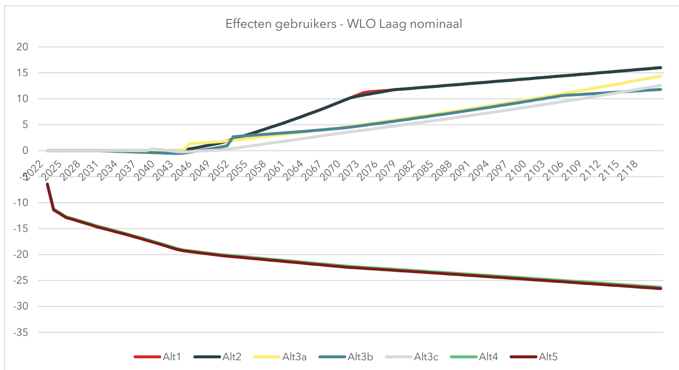
Figuur B.8 Tijdreeks effecten gebruikers in WLO-Laal in nominale waarden (mln. euro's) ten opzichte van het nulalternatief over zichtperiode MKBA
