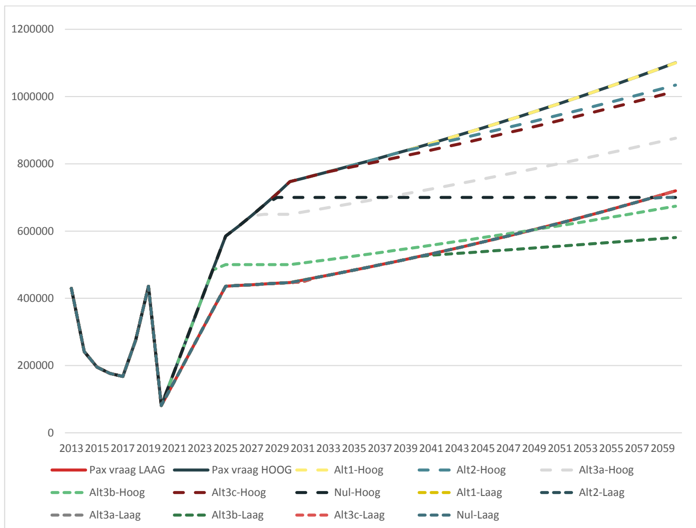
Figuur 2.3 Ontwikkeling passagiersvolumes (aantal passagiers) per alternatief 15
