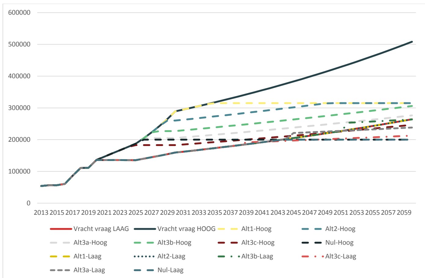
Figuur 2.2 Ontwikkeling vrachtvolumes in tonnages per alternatief 14
